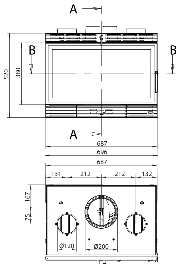
B-B
