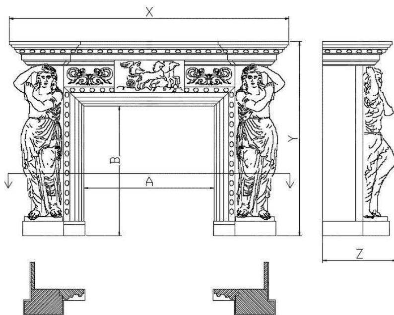
SECCIÓN A-A'
