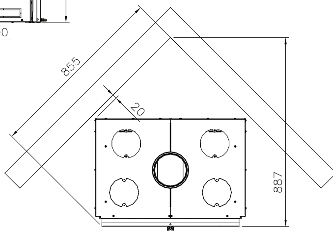
INSERTO 70 WIDE
