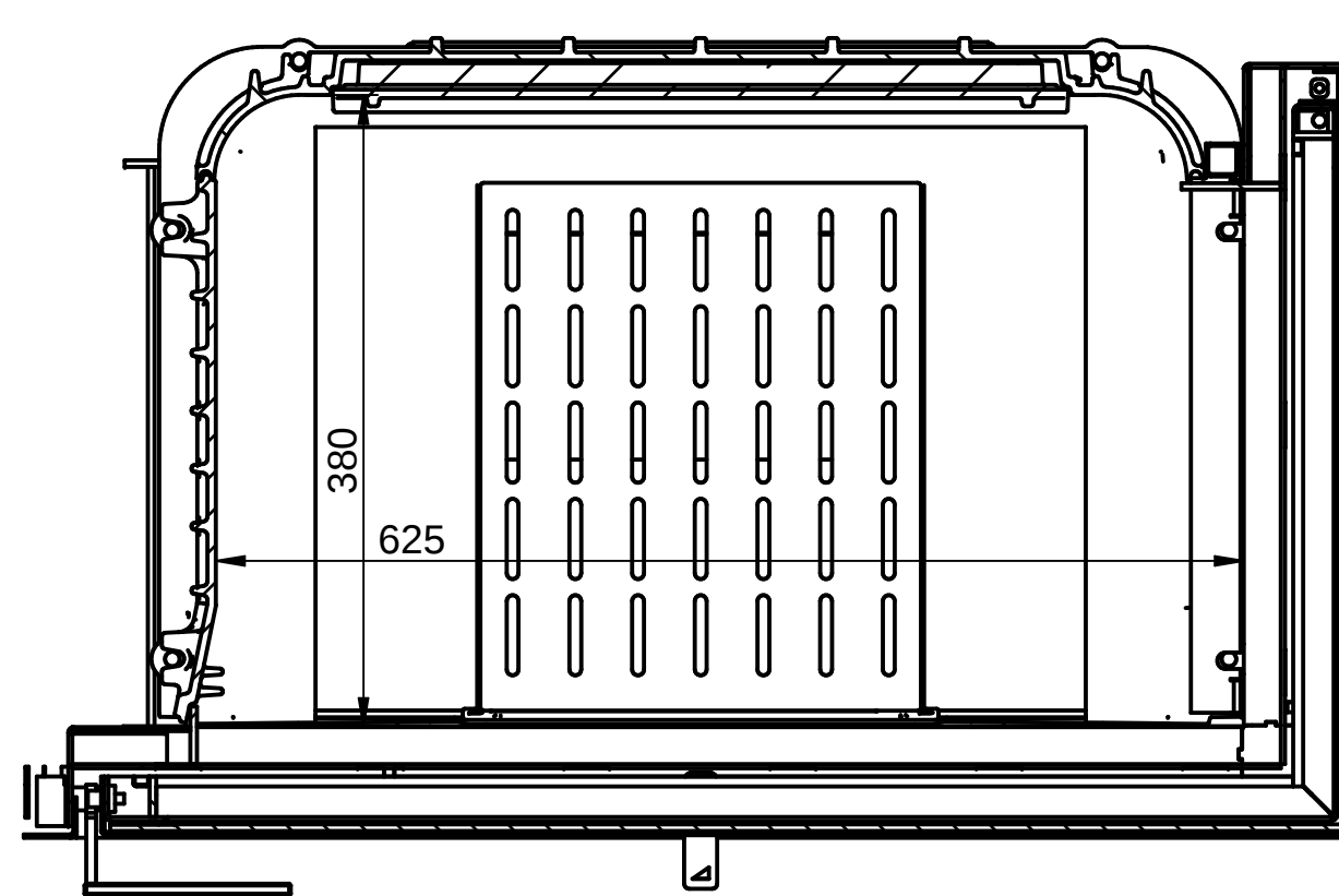
SECTION A-A
