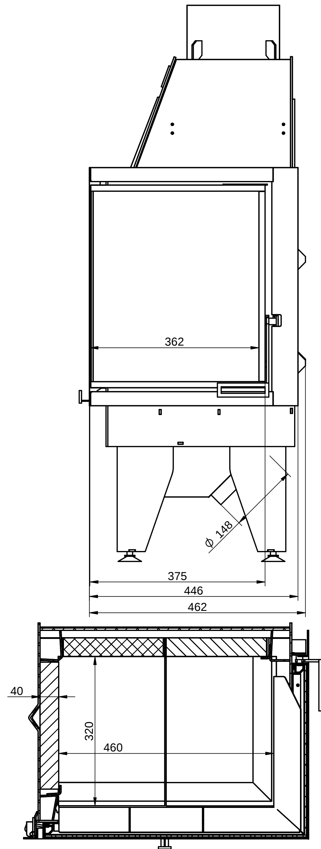
SECTION A-A
