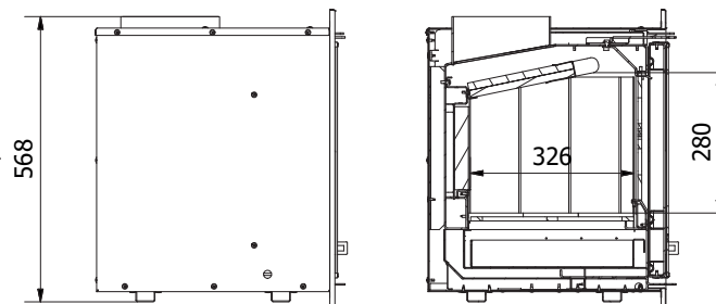
A-A
