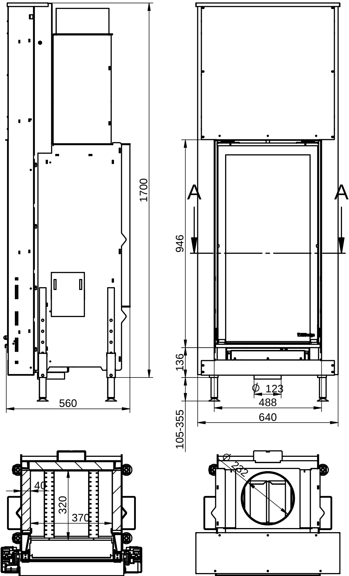
SECTION A-A
