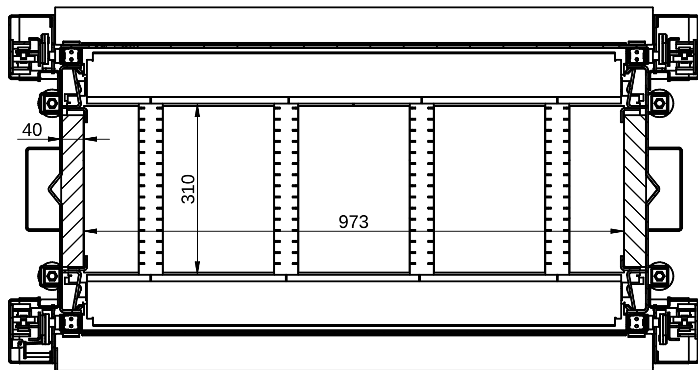
SECTION A-A
